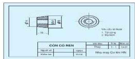
Hình 7.2.1. Bản vẽ chi tiết côn có ren
